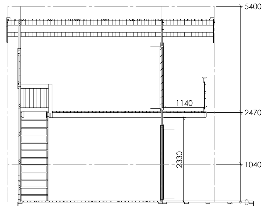
C-C 1
