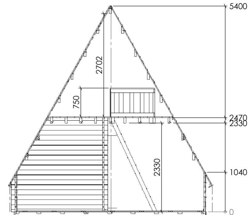
C-C 2
