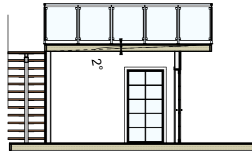
Sektion B-B
