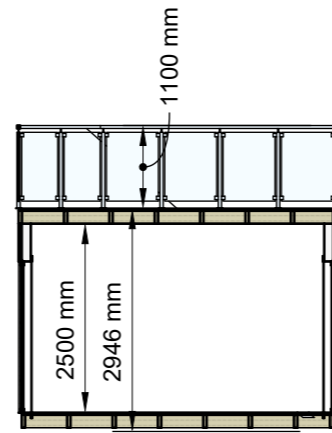
Sektion A-A
