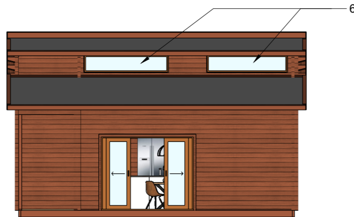
Fasad framifrån
