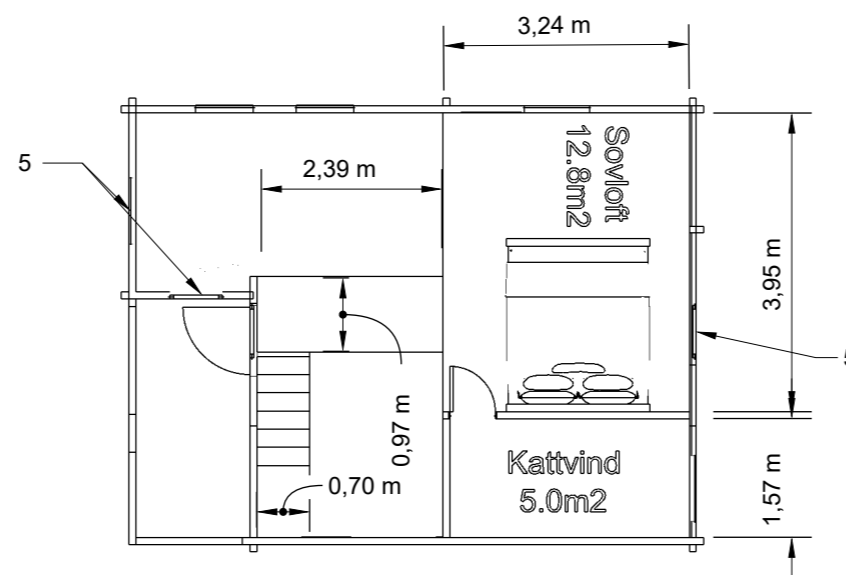
Loftplan
