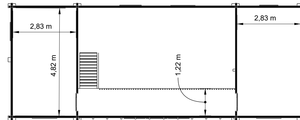
Loftplan
