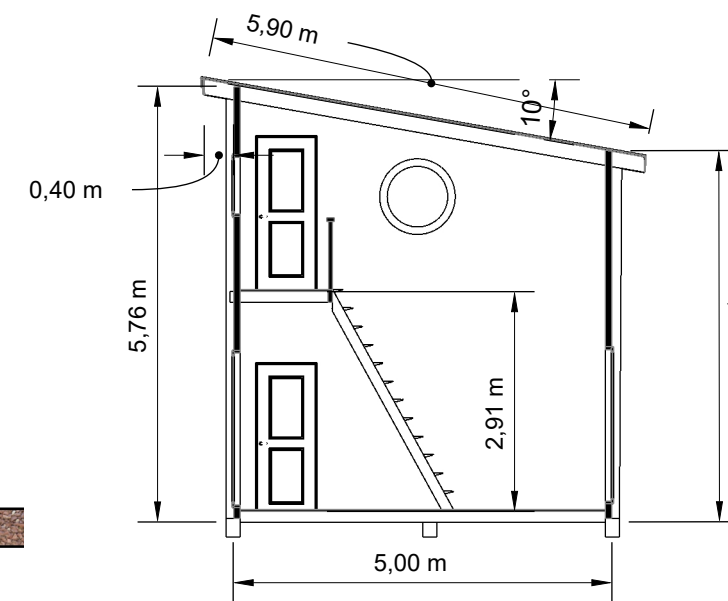
Sektion
